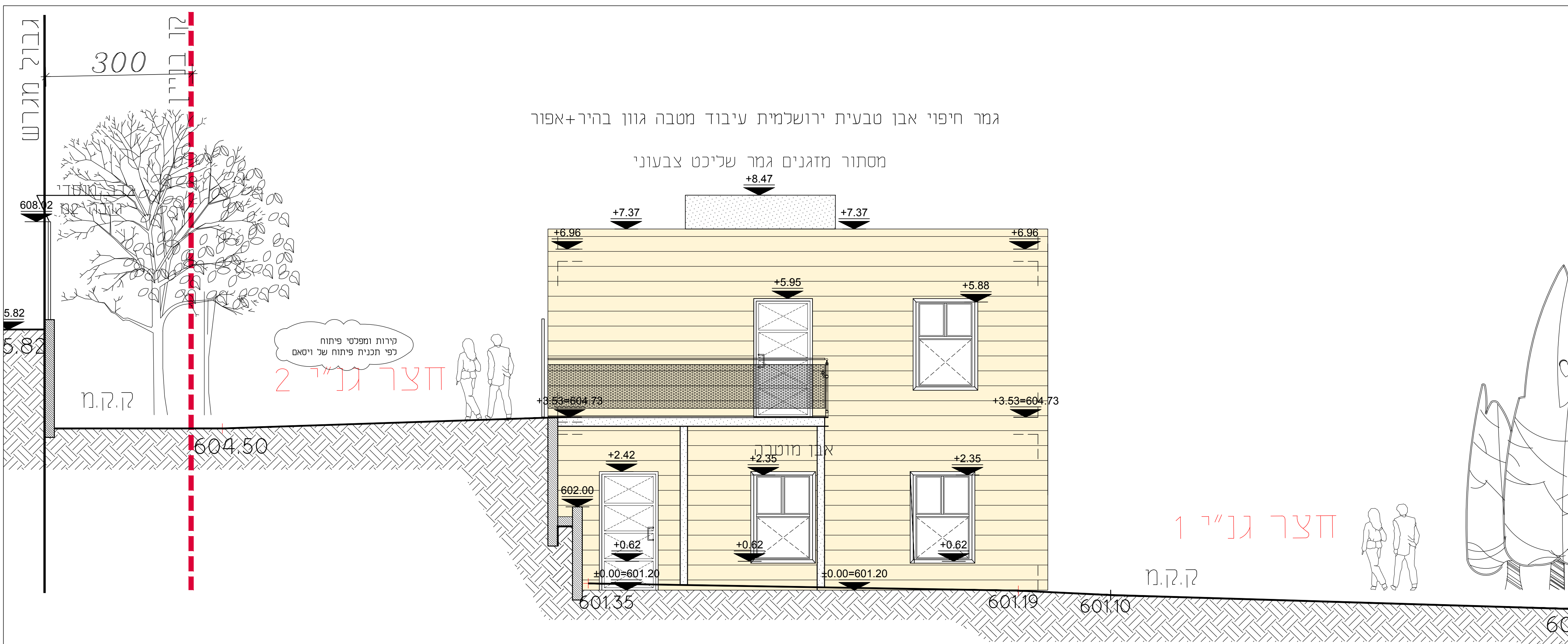
חזית מזרחית (4) קנ"מ 1:50
